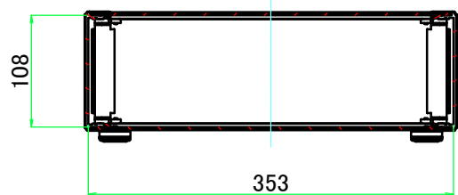
A-A ( 1 : 6.5 )
