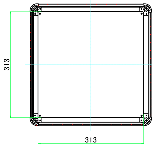
C-C ( 1 : 6.5 )
